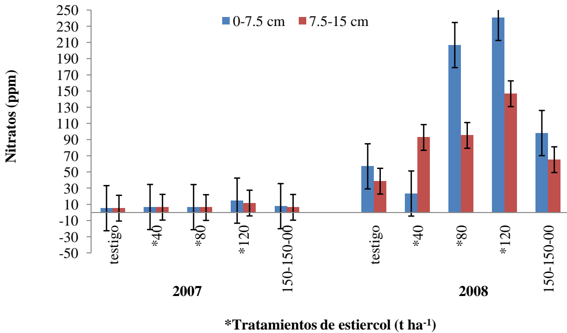
Figura 8. Contenido de Nitratos en el suelo (ppm), en dos profundidades y dos años de estudio, en los diferentes tratamientos de estiércol solarizado. CAE-FAZ-UJED, 2007- 2008.
